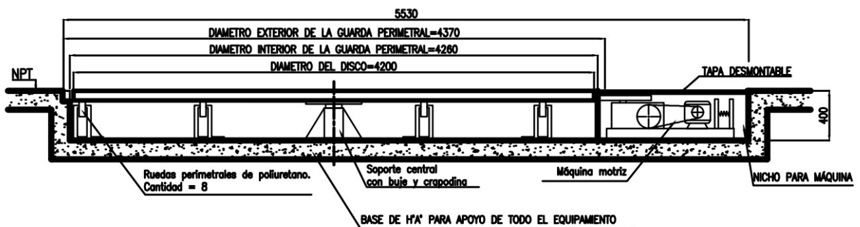
CORTE A-A ESCALA 1 : 20
