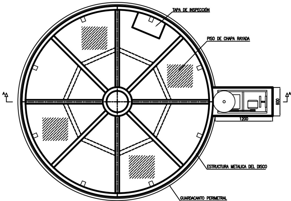
VISTA EN PLANTA ESCALA 1 : 20
